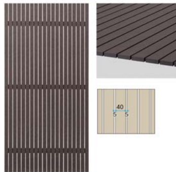
密縦板貼 40幅
