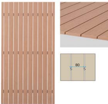
密縦板貼 80幅
