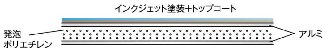
【エバーアートボード®シックシリーズ ボード断面図イメージ】
